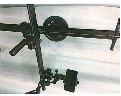
Z軸レール及びX-Y軸レール モバイルグラケット
